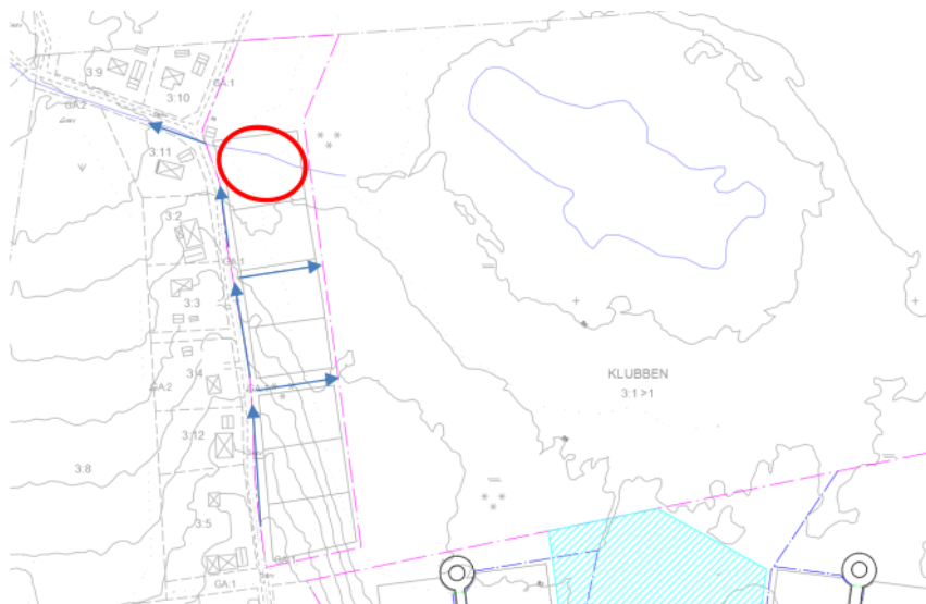
Figur 21. Förslag på dikes- och åtgärdsplacering med rinnpilar i det norra området. Den röda ringen visar lokalisering för en bäck som kopplar samman Lomtjärnen med Bjännsjön och som lämnas orörd utanför planområdet. Källa: Sweco
