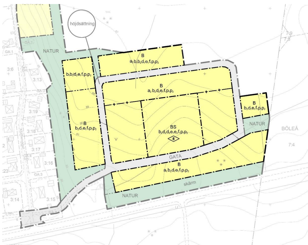
Figur 9. Urklipp ur plankarta över bebyggelseområden i den södra delen av planområdet. Källa: Sweco
