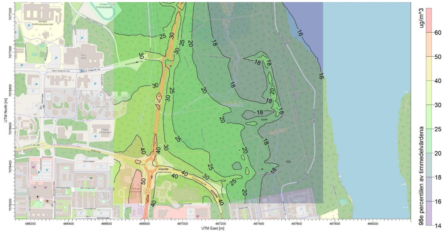
Figur 5, 98e percentilen av timmedelvärdet av NO 2 . Varje linje på kartan motsvarar en beräknad halt, i det färgade området mellan två linjer är halten mellan linjernas värde. Gränsvärdet i MKN är 90 µg m -3 .
