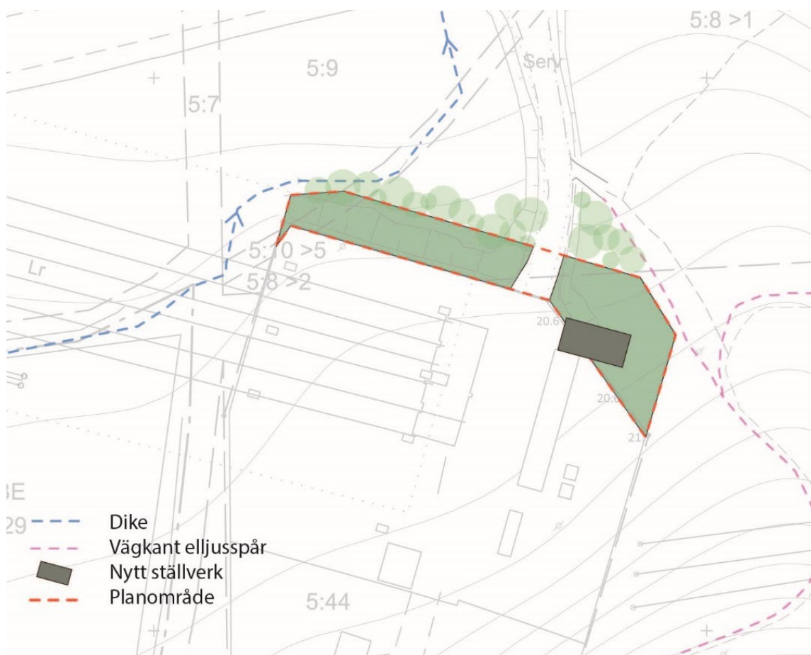
Figur 13. Situationsplan som visar möjlig placering av den tillkommande byggnaden gällande 12 KV ställverket samt hur planförslaget förhåller sig till befintligt elljusspår och dike.
